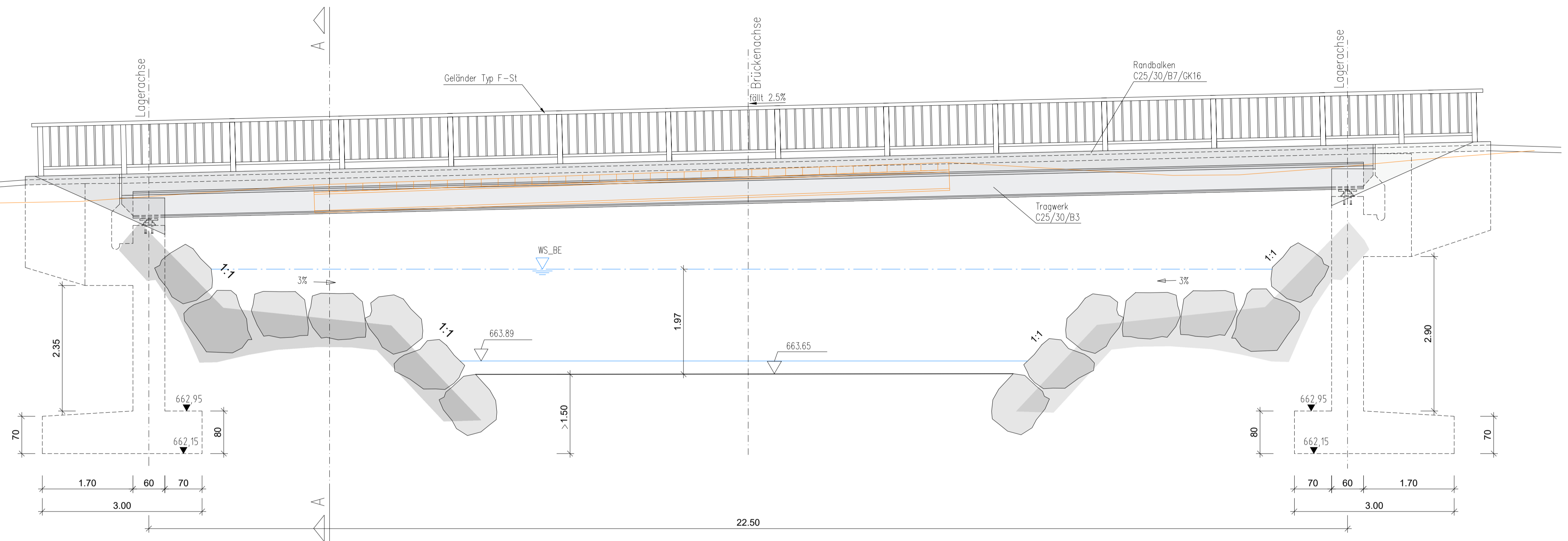
Ansicht C-C Tragwerk M 1:50
