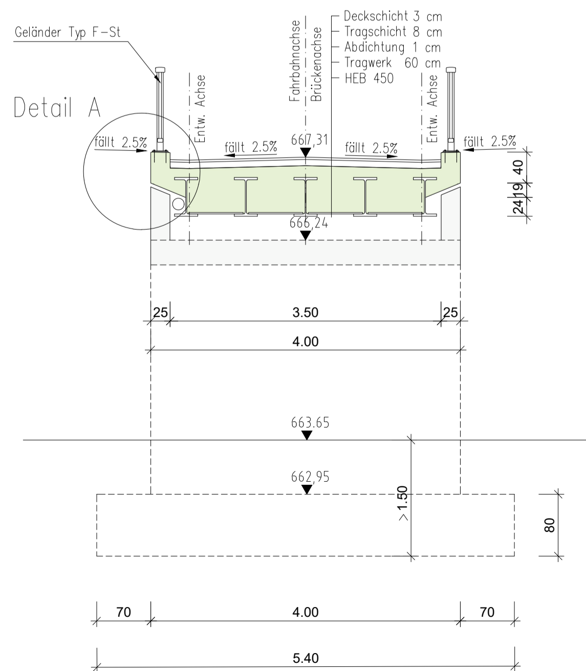
Schnitt A-A Tragwerk M 1:50
